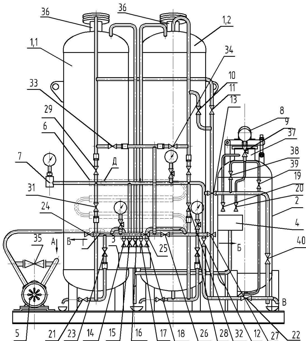
Рис.2- Блочная водоподготовительная установка ВПУ-10,0 У-М.
